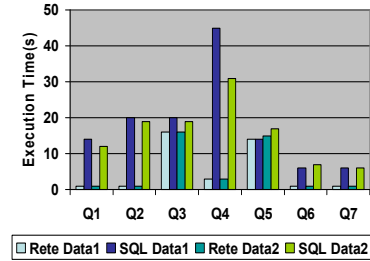
Fig. 4. Execution Times of Q1-Q7
